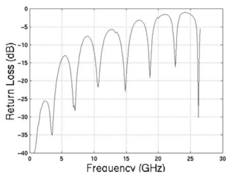
S_{11} du premier câble avec connecteur droit
