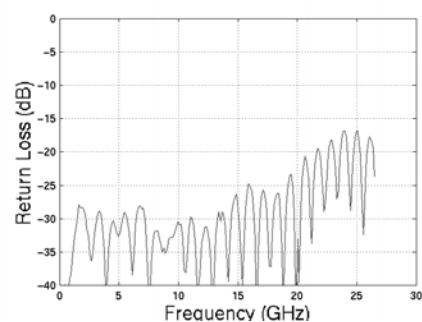
S_{11} du cable avec connecteur coudé
